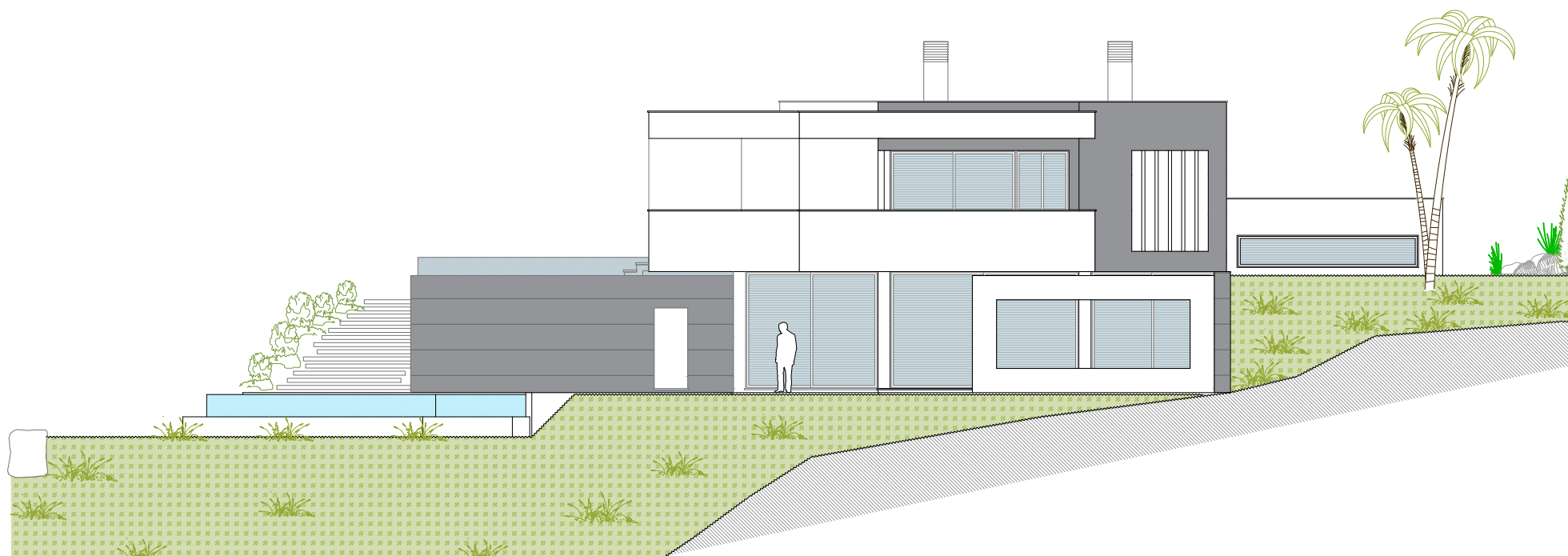
ALZADO NORTE
