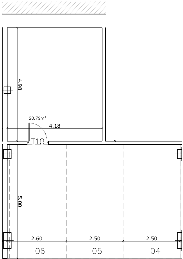
APARCAMIENTOS Y TRASTERO
